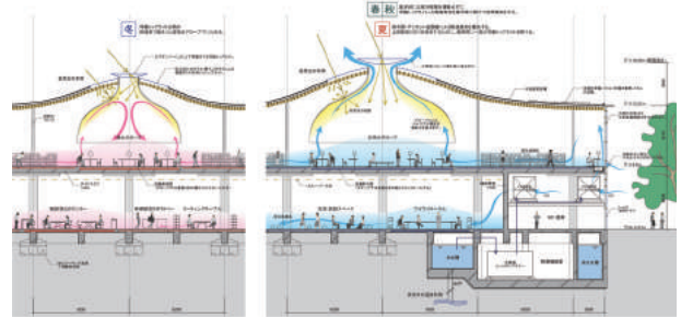
みんなの森 ぎふメディアコスモス 環境ダイアグラム
